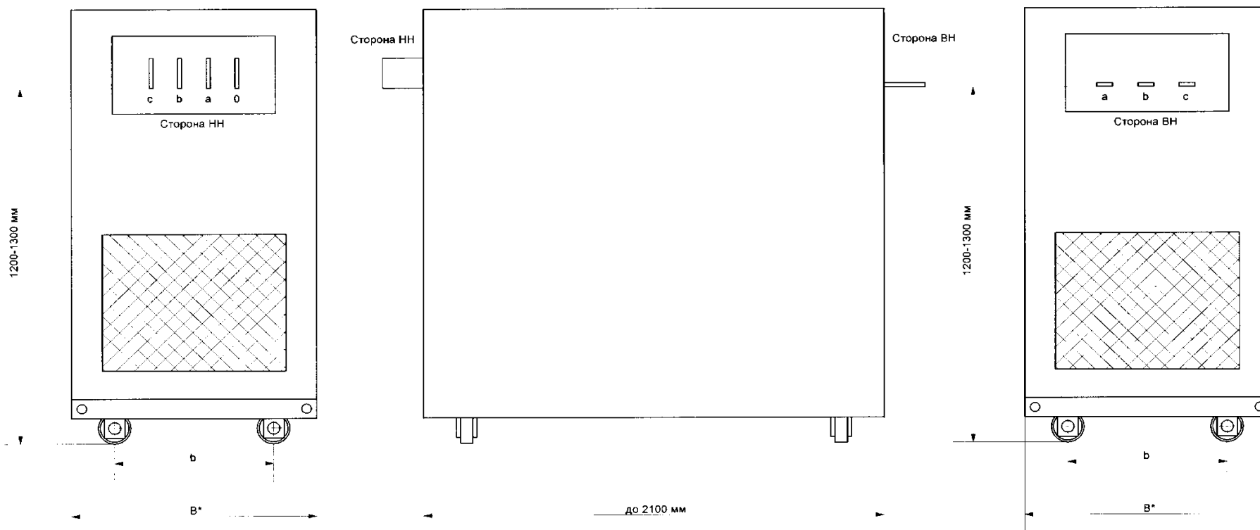
Основные габаритные и присоединительные размеры трансформатора с кожухом на 500 кВА
